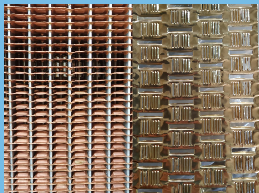
串片式铜水箱芯体
