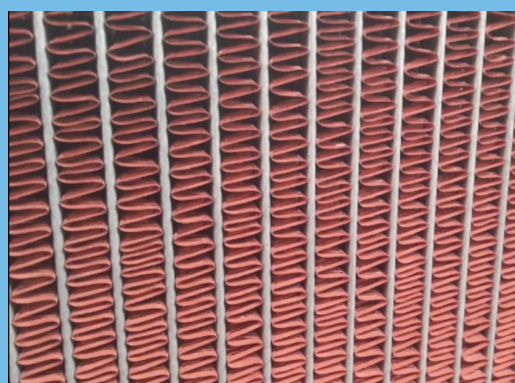
摆带式铜水箱芯体
