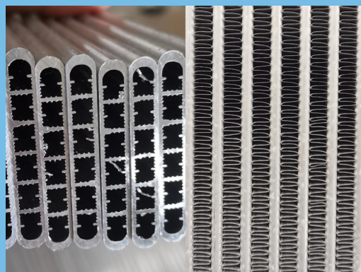
摆带式油散芯体
