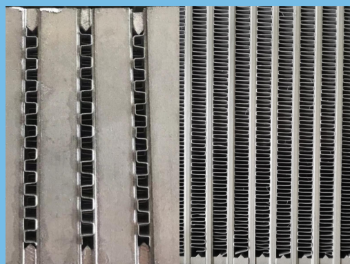
串片式铝水箱芯体
